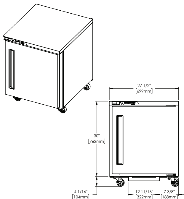
ELEVATION
